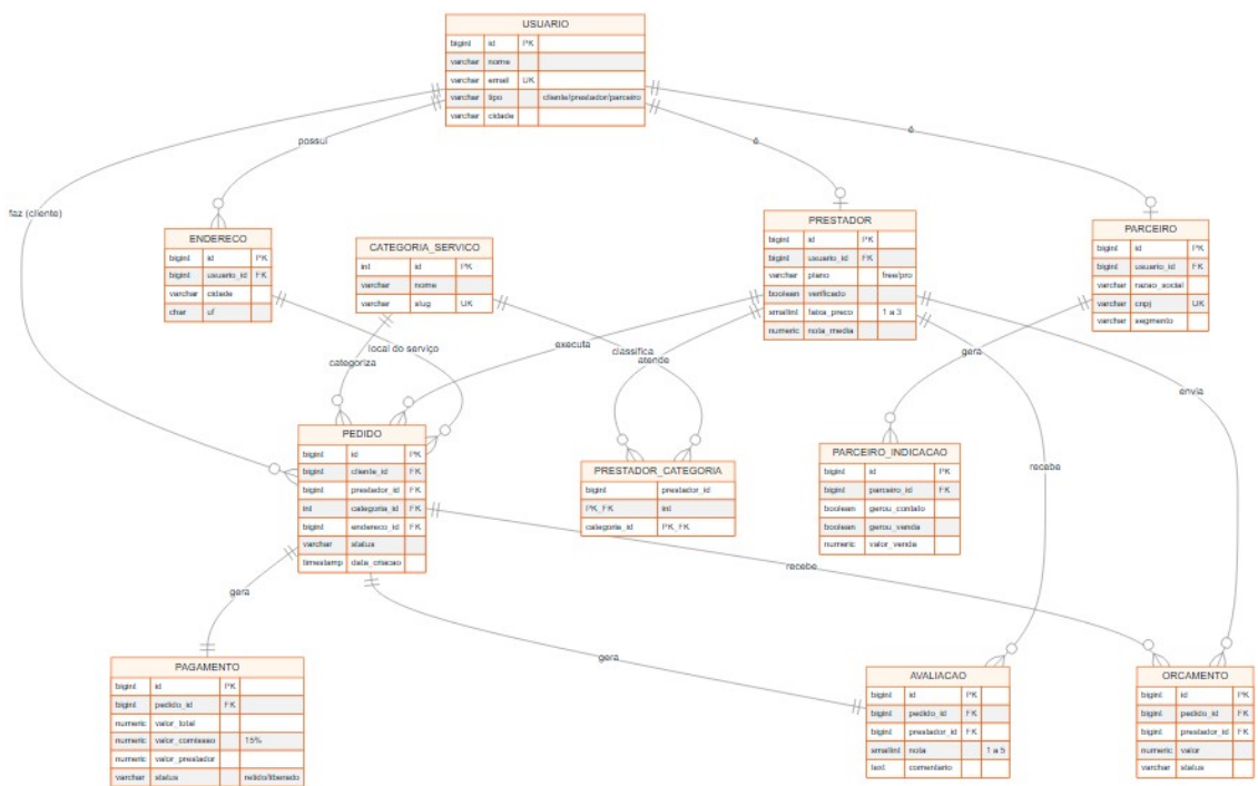
Figura 2 — Diagrama Entidade-Relacionamento do banco transacional (OLTP).
