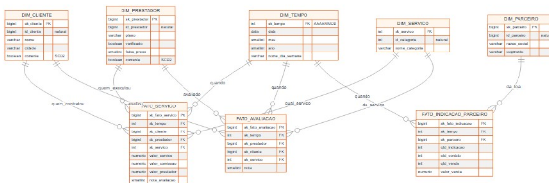
Figura 3 — Esquema estrela do Data Warehouse (constelação de fatos).
